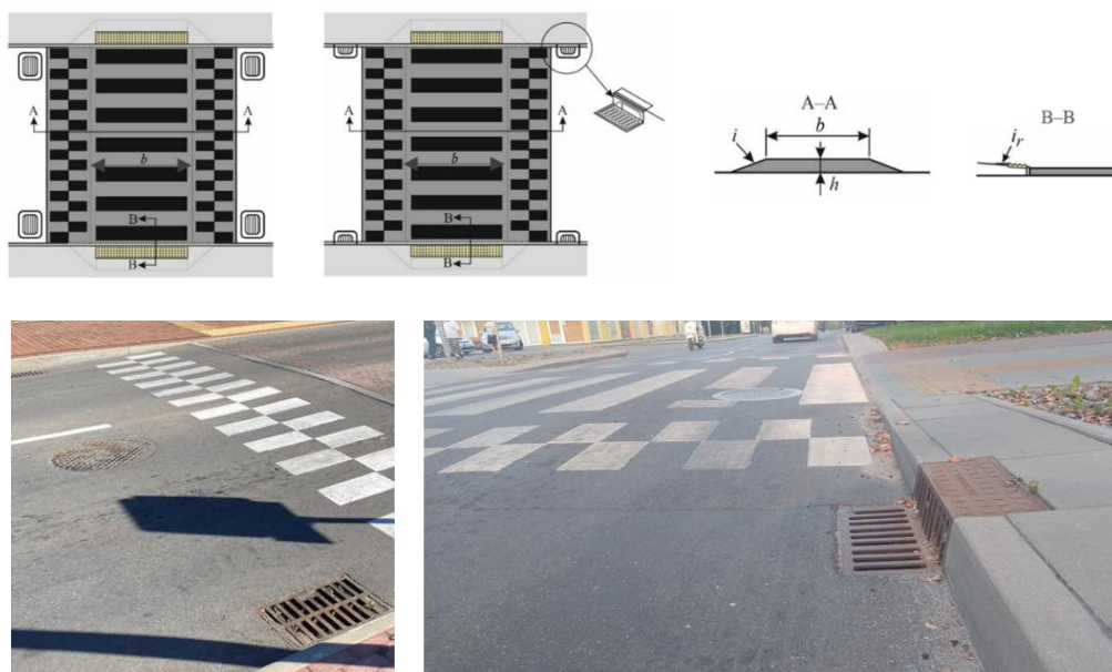
pav. 7.5 Iškiliosios pėsčiųjų perėjų schemas ir pavyzdys (su lietaus vandens nuleidimo sprendiniais)
