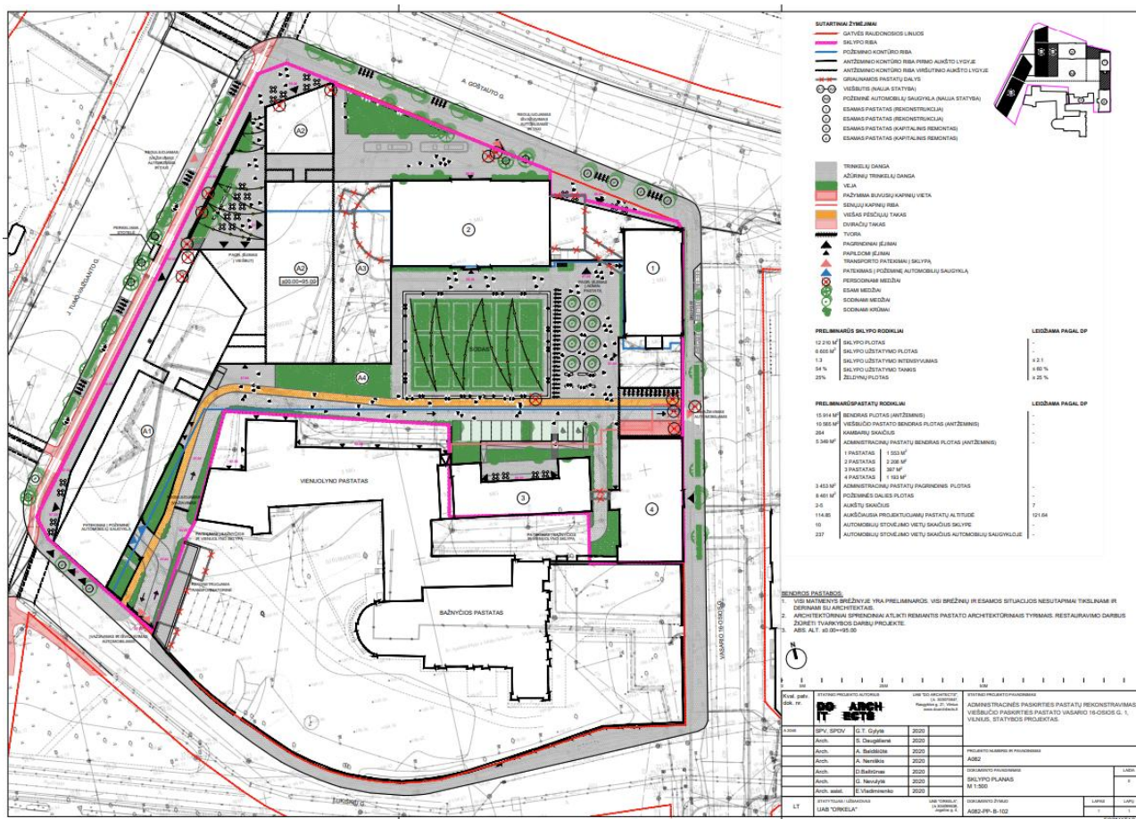
pav. 7.9 UAB „DO ARCHITECTS“ projektinių pasiūlymų brėžinio iškarpa. Projekto numeris: A082
