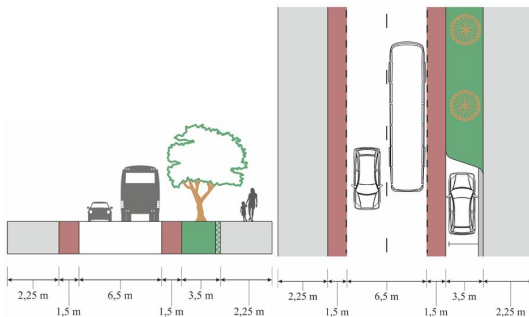
pav. 7.1 \leq 30 km/h greičio režimo gatvės skersinis profilis su maršrutinio transporto eismu
