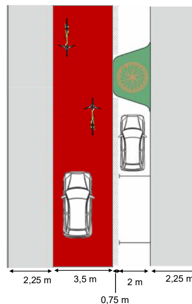
Pjūvis 6 – Vienpusis eismas su parkavimu vienoje gatvės pusėje ir šaligatviais abejuose gatvės pusėse:
