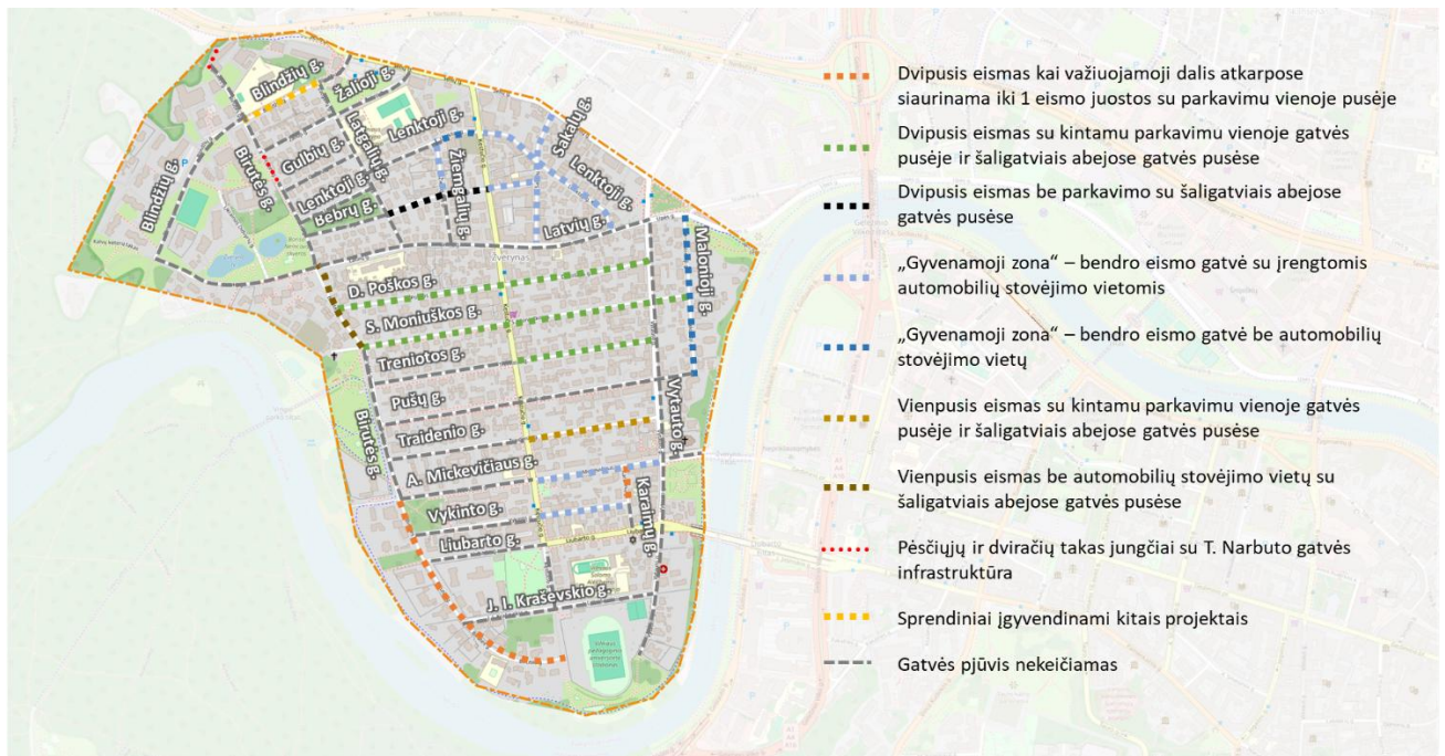
pav. 8.3 Pirmosios alternatyvos gatvių erdvių pertvarkymo sprendiniai
