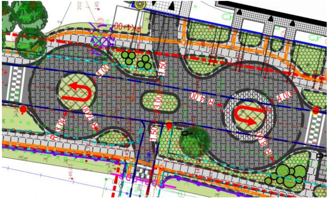
pav. 8.14 Gatvės pertvarkymo pavyzdys, kai suformuojami aklakeliai motoriniam transportui, bet paliekama galimybė pravažiuoti bevarikliam ir specialiajam transportui
