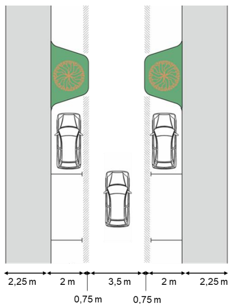
Pjūvis 7 – Dvipusio eismo dviračių gatvė su parkavimu ir šaligatviais abejuose gatvės pusėse:
